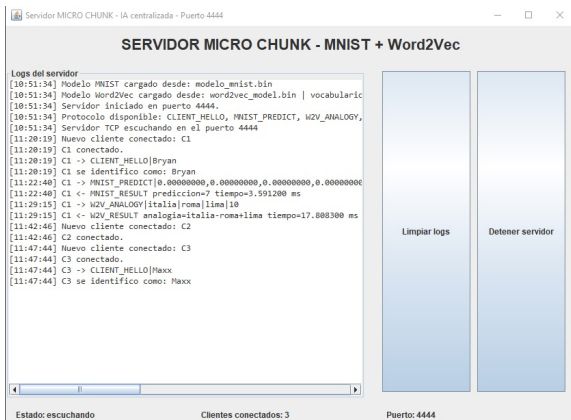
Figure 12: Servidor atendiendo múltiples hilos/lenguajes en paralelo
